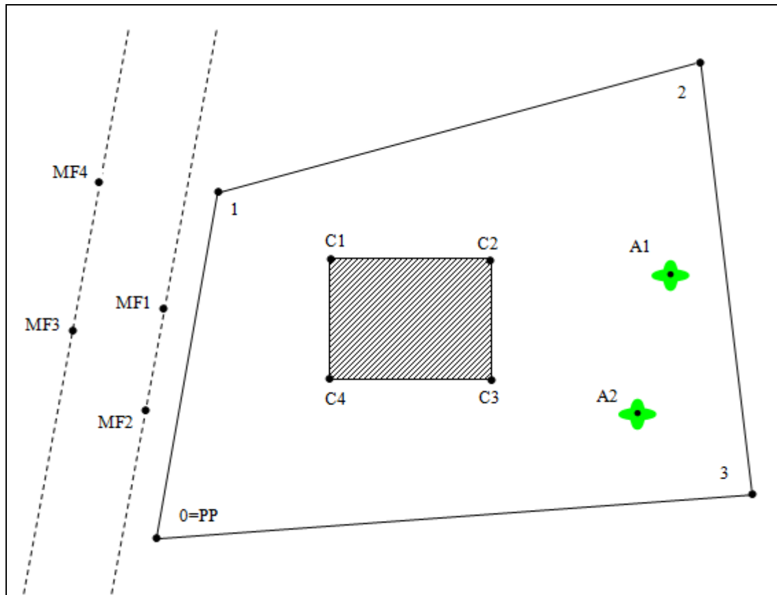
Figura 1 – Croqui de poligonal fechada e detalhes.
